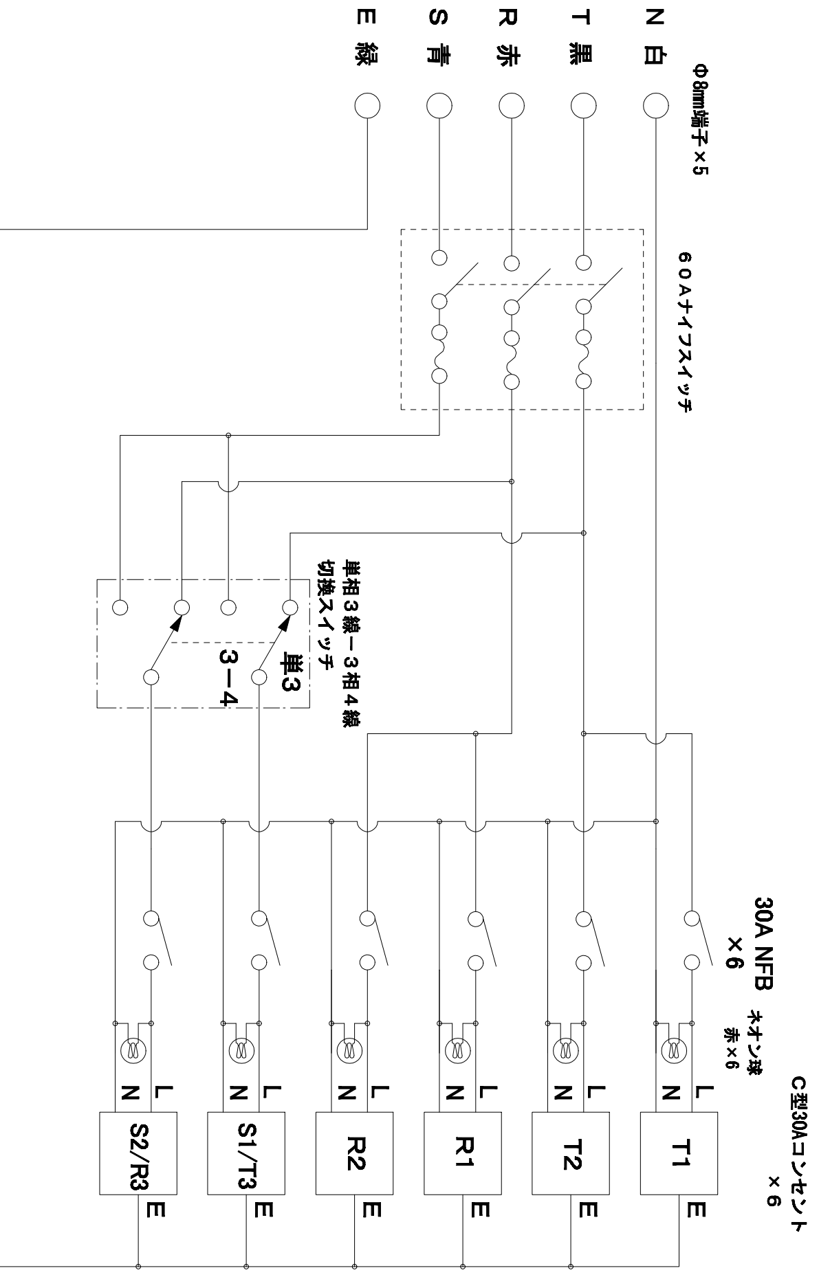
コンボックス CB-601 回路図
